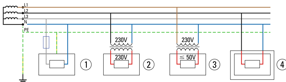
Die vier latenten Schutzmassnahmen gegen elektrischen Schlag nach NIN 4.6
